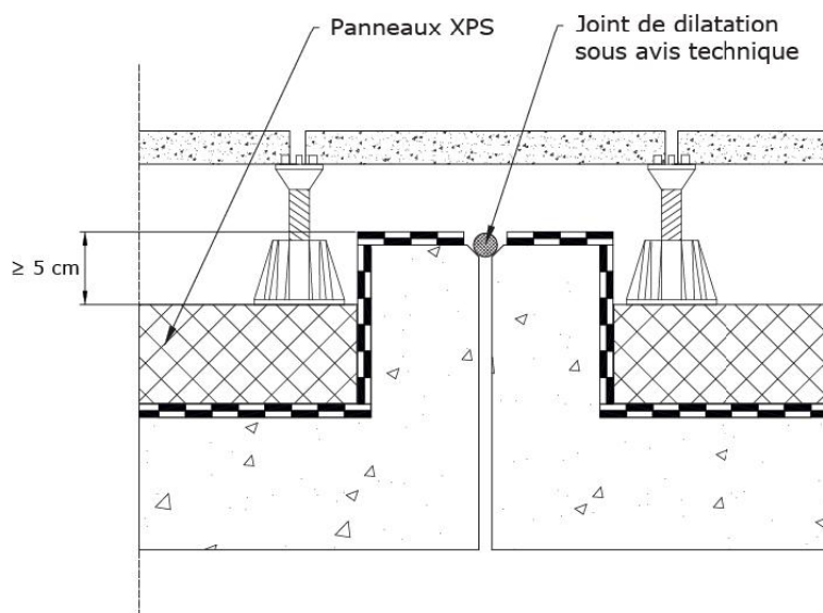
Figure F.6 - Toiture-terrasse accessible aux piétons avec protection par dalles sur plots - Joint plat surélevé - Exemple
