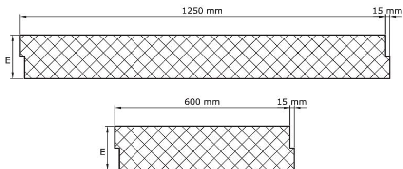
Figure F.1 - Vue en coupe d'un panneau XPS type
