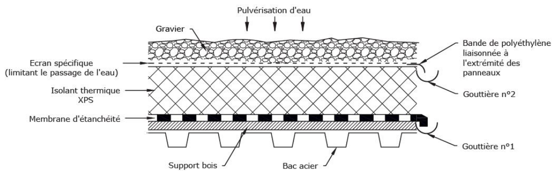
Figure E.2 - Schéma en coupe du montage
