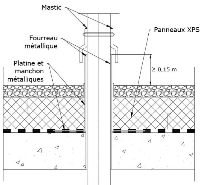
Figure F.7 - Traversée de ventilation - Exemple de solution
