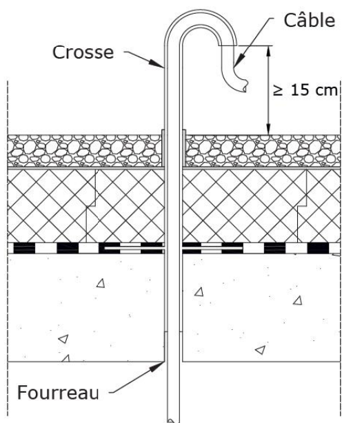
Figure F.8 - Passage de câble d'alimentation - Exemple de solution
