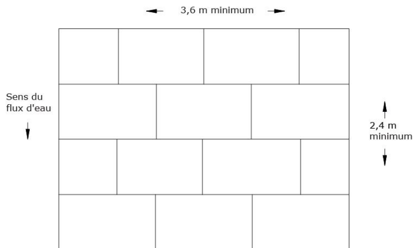
Figure E.1 - Exemple de positionnement des panneaux
