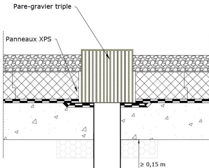
Figure F.9a ter - E.E.P. - Toiture inaccessible - Exemple de solution - Variante 2
