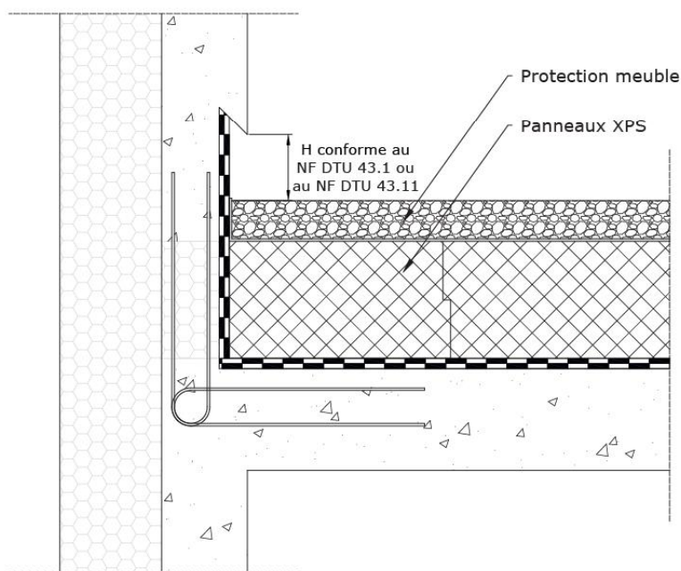
Figure F.2a - Toiture-terrasse inaccessible - Isolant XPS - Pose en un lit - Exemple
