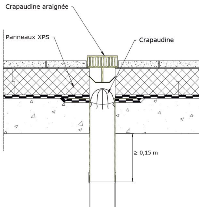
Figure F.9b - E.E.P. - Toiture technique - Exemple de solution
